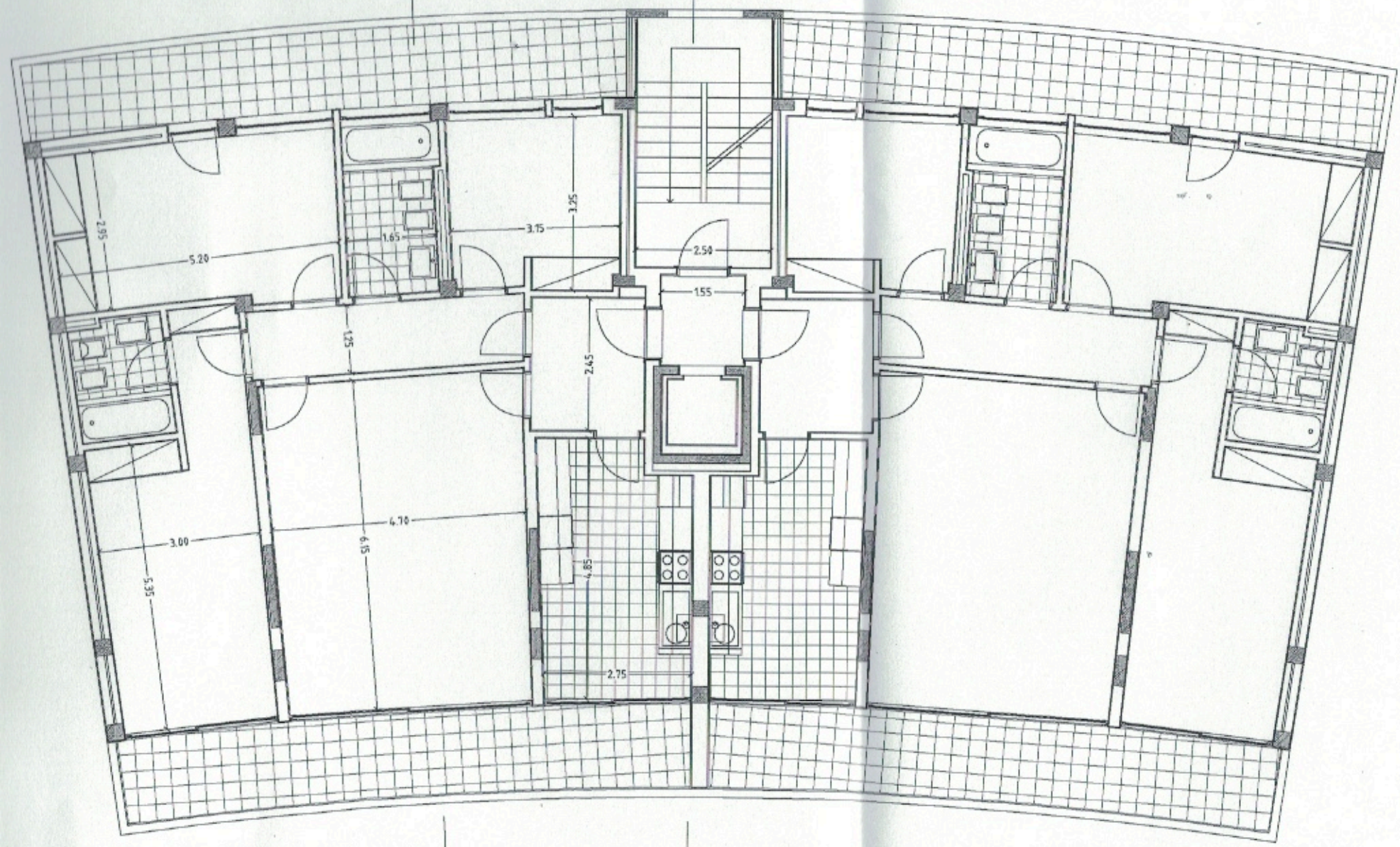
Planta - 1º Andar
