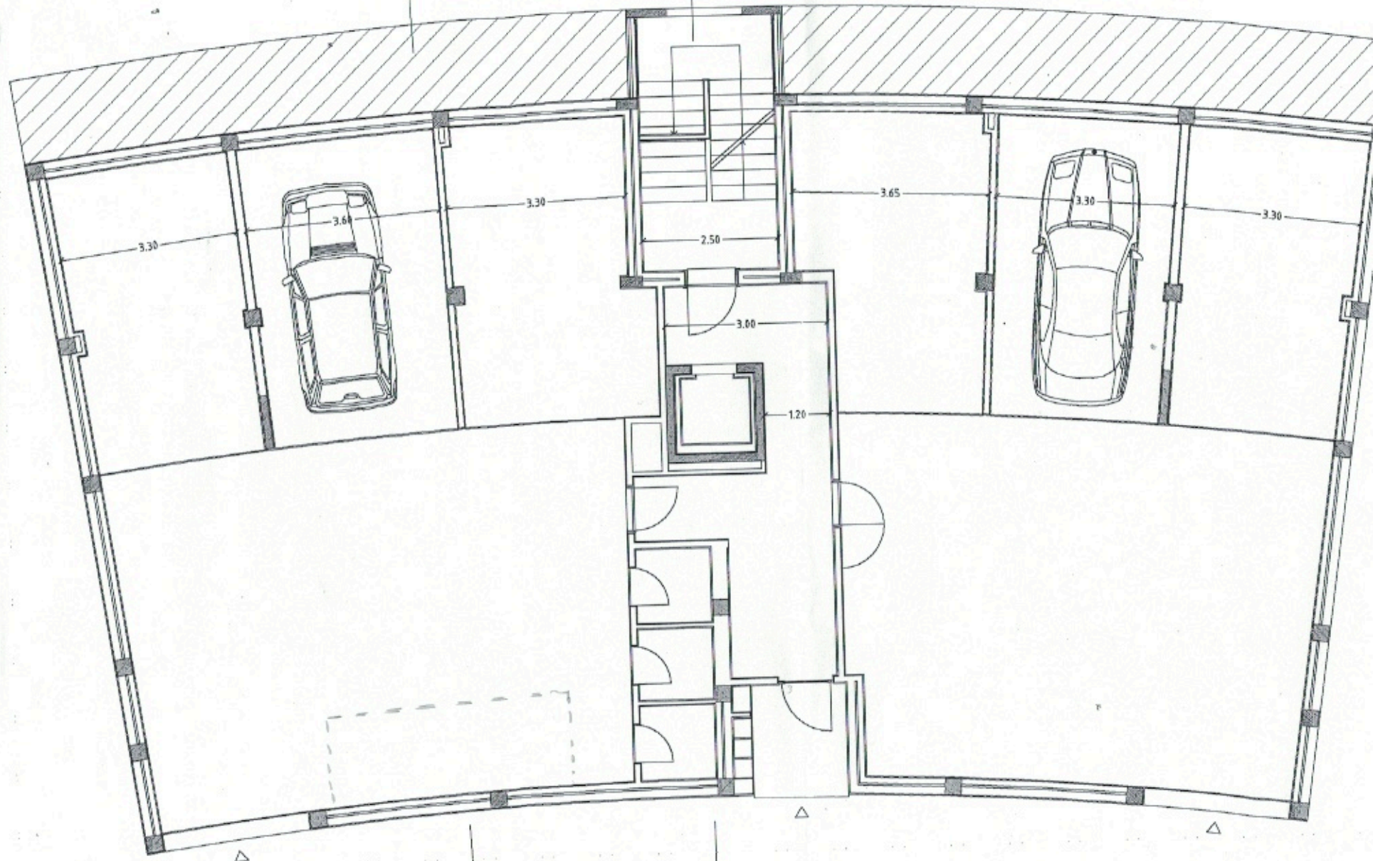
Planta - Rés do Chão
