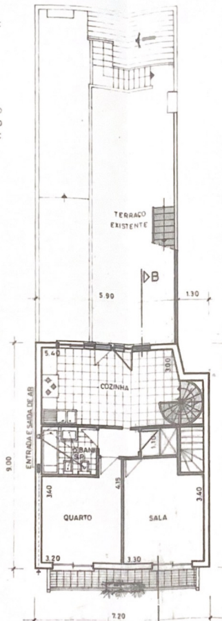
1º ANDAR a construir
