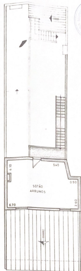
COBERTURA E SOTÃO
