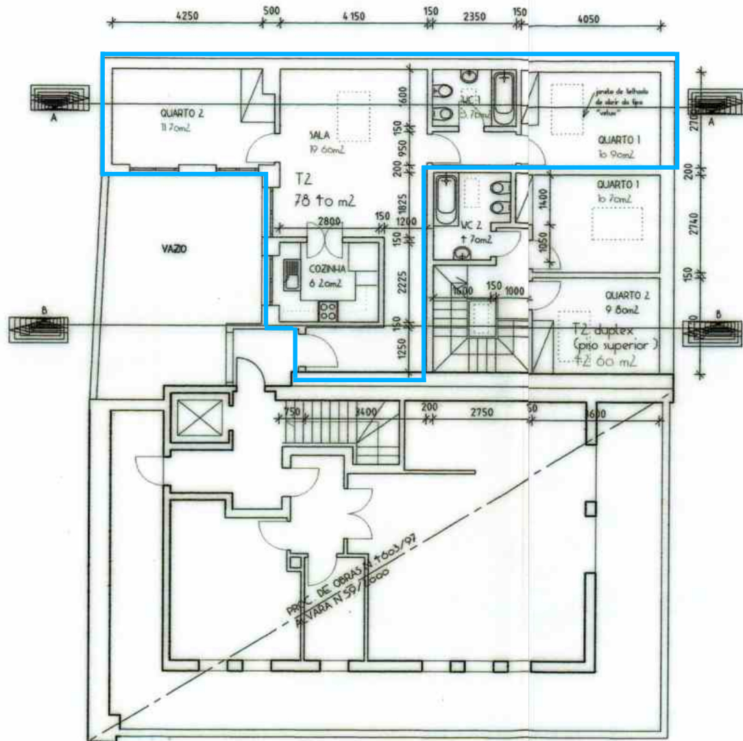
PLANTA FINAL DO PISO 3 escala 1 : 100
